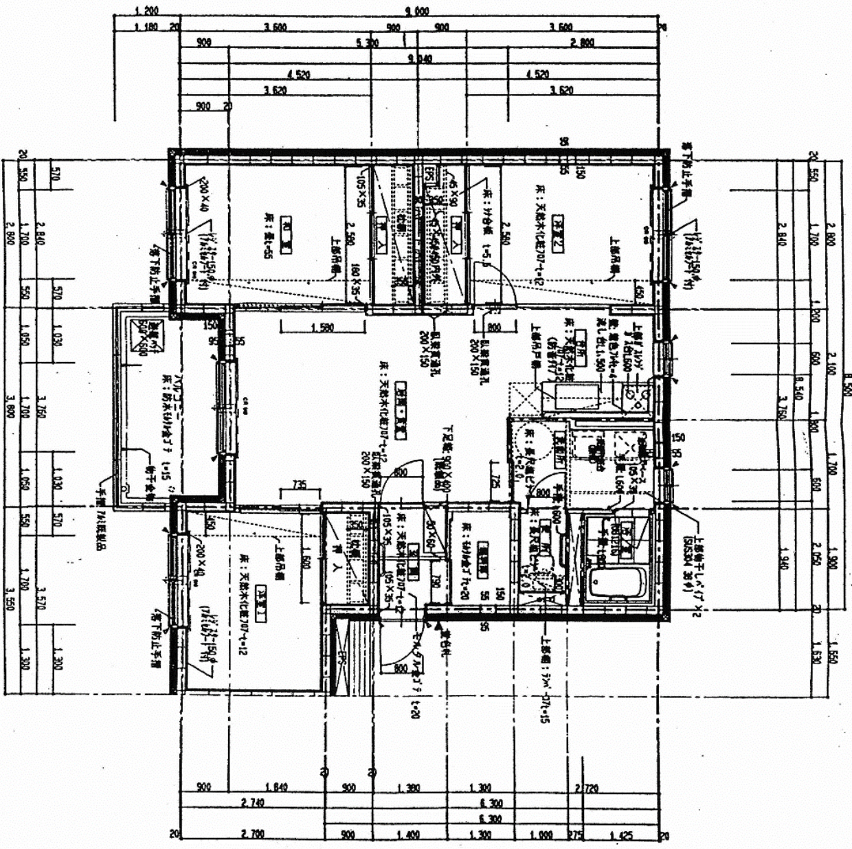
平面詳細圖
